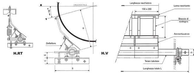
BRACCI DI SOSTEGNO - DIMENSIONI A e H
